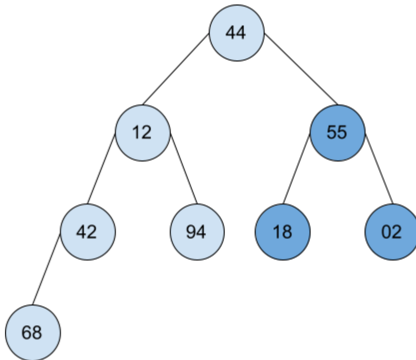
Subárvore Raiz 55
